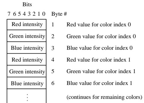
Fig. 3.14: GIF color map.
