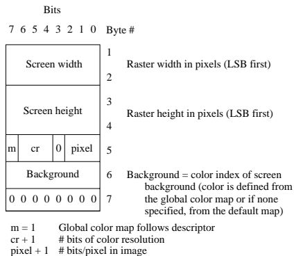
Fig. 3.13: GIF screen descriptor.
